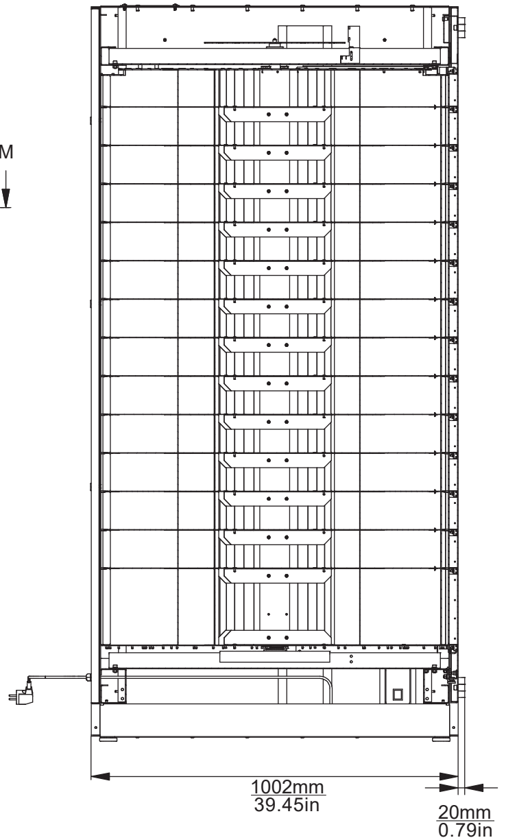
A-A ( 1:10 )
