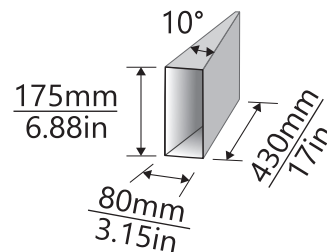
TYP B4
